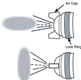
(Dwg. TP2053)
