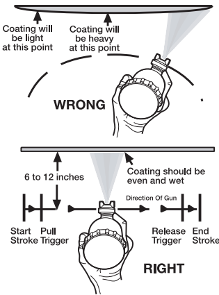
(Dwg. TP2049)
